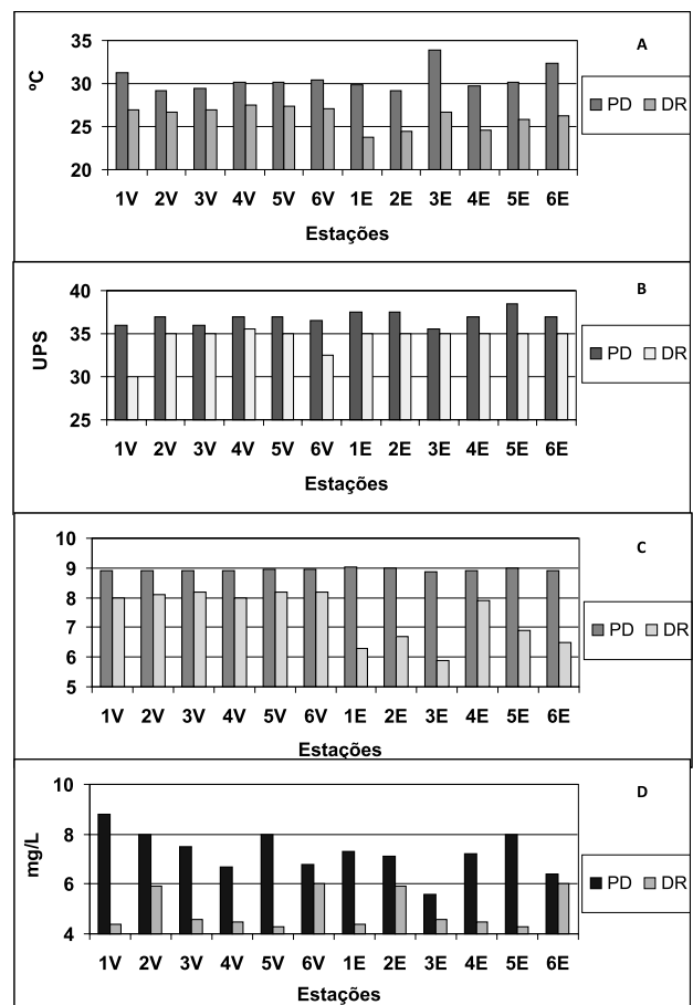
Figura 3 - Temperatura (A), salinidade (B), pH (C) e oxigênio dissolvido (D), na Pré-dragagem (PD) e Dragagem (DR), no Porto de Aratu, Baía de Todos os Santos, Bahia. (V, vazante; E, enchente).
