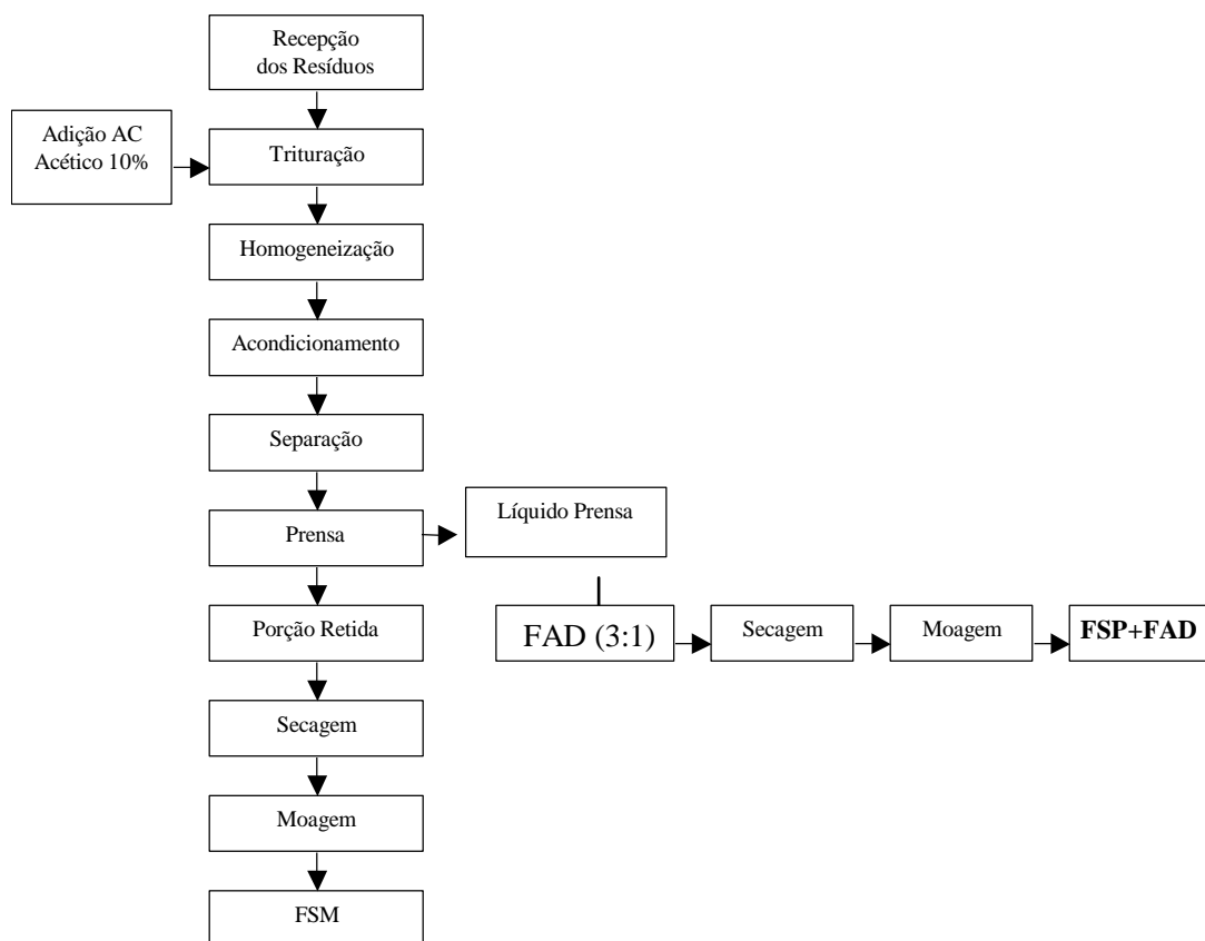
Figura 1: Fluxograma de obtenção da farinha de silagem mais farelo de arroz desengordurado.
