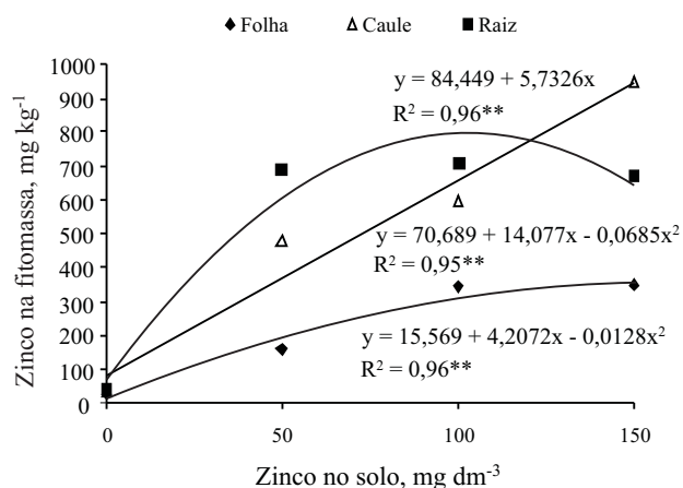
Figura 7 - Teores de zinco nas folhas, caule e raízes do pinhão-manso em função das doses de zinco aplicadas ao solo
