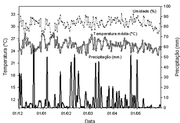
Figura 1 - Variação diária da umidade, temperatura média do ar e precipitação pluvial de novembro de 2007 a maio de 2008, UFT, Palmas - TO Fonte: INMET, 2008. (Estação Climatológica de Palmas - TO)
