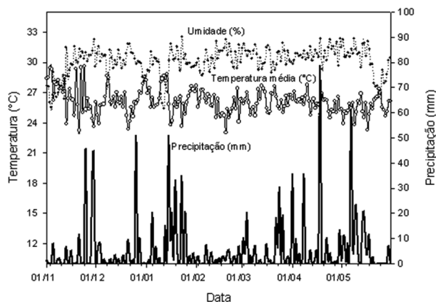
Figura 2 - Variação diária da umidade, temperatura média do ar e precipitação pluvial de novembro de 2007 a maio de 2008, UFT, Gurupi - TO Fonte: INMET, 2008. (Estação Climatológica de Gurupi - TO)
