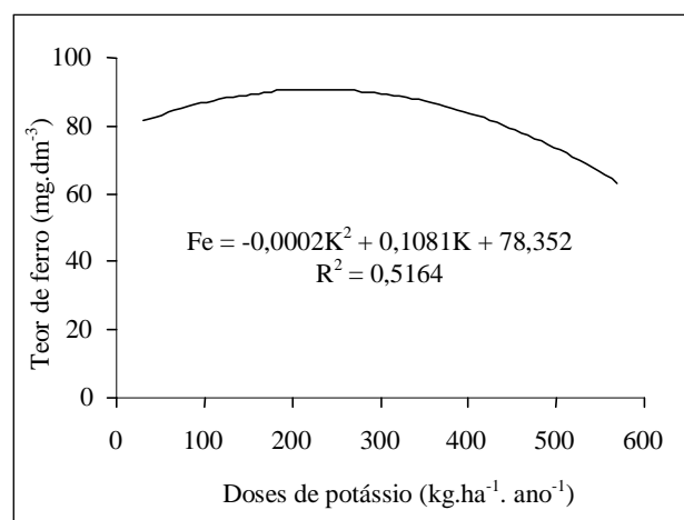
Figura 2 – Teor de ferro no solo na profundidade de 0,0 a 0,2 m em função das doses de potássio aplicadas no solo via água de irrigação.
