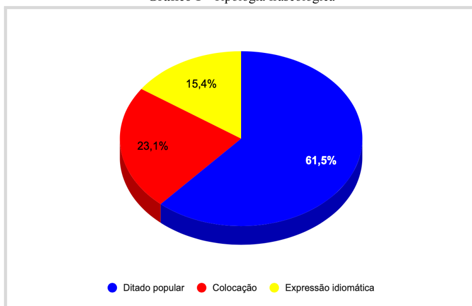
Gráfico 1 - Tipologia fraseológica
