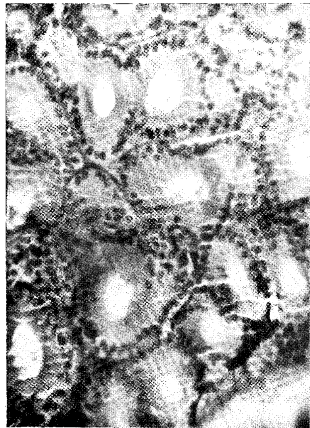
Figura 1 — Microfotografia (X120) de um corte histológico de testículo de Panulirus laevicauda (Latr.) no estágio I — estágio inicial.
