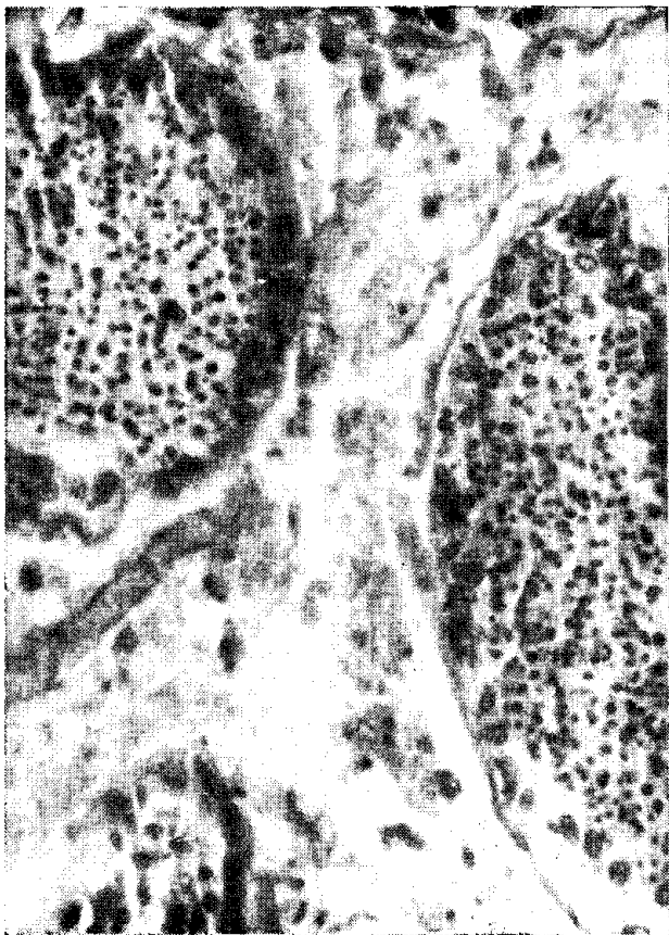
Figura 2 — Microfotografia (X240) de um corte histológico de testículo de Panulirus laevicauda (Latr.) no estágio II — estágio de desenvolvimento.
