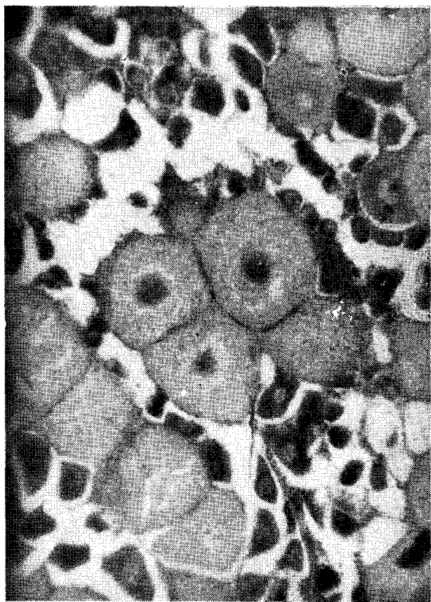
Figura 7 — Microfotografia (X 120) de um corte histológico de ovário de Panulirus laeviscauda (Latr.) no estágio III — estágio de pré-maturação.
