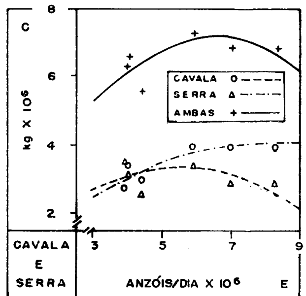
Figura 2 — Curvas de rendimento da cavala, Scomberomorus cavalla (Cuvier), e da serra, Scomberomorus maculatus (Mitchill), em separado e em conjunto, nas águas costeiras do Estado do Ceará (Brasil).
