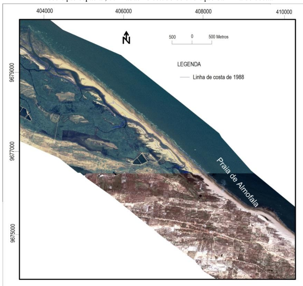
Figura 3: Mosaico de imagens multiespectrais do satélite Quickbird do ano de 2004, que possuem alta resolução espacial, utilizadas no estudo de evolução da linha de costa.
