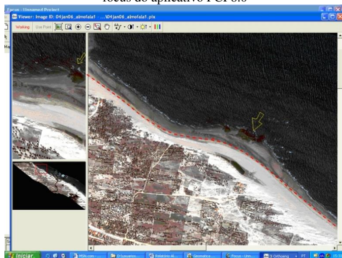
Figura 4: Linha de costa (2004) e plataforma de abrasão da praia de Almofala (seta), em zoom no focus do aplicativo PCI 8.0
