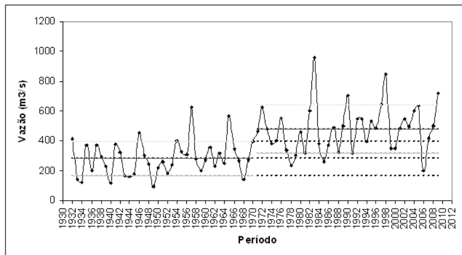
Figura 2 – Períodos hidrológicos – PH – da estação fluviométrica de Jatatizinho 64507000. Linha vermelha: média. Linha amarela: +1 SD e Linha verde: -1 SD. Ponto vermelho: Fechamento das comportas da UHE Capivara, localizada no médio Paranapanema.
