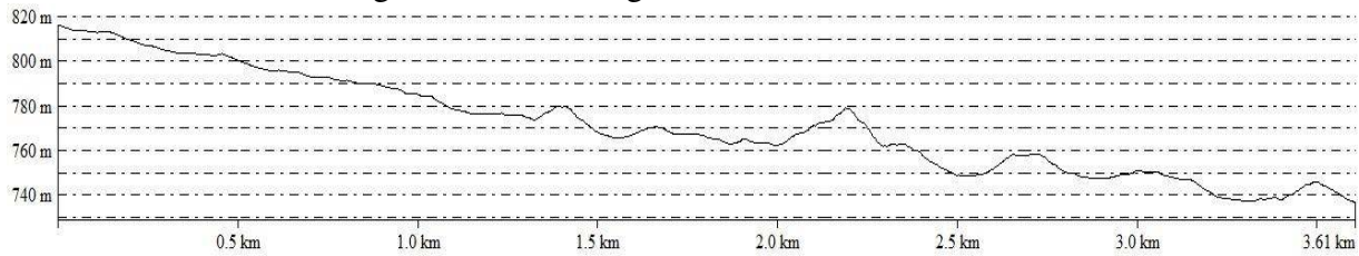
Figura 4 - Perfil longitudinal do riacho de Vila Maria
