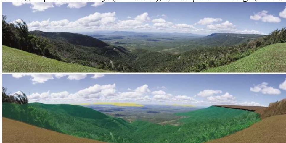
Figura 3 – Visualização de feições geomorfológicas do Mirante: topo do Glint da Ibiapaba (filtro marrom); zona de escarpa (preto); superfícies soerguidas e pedimentos dissecados (filtro verde); Depressão Sertaneja (cor natural); e, maciços e inselbergs (filtro amarelo)
