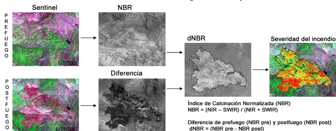
Figura 4 – Flujo de trabajo para la estimación del Índice de Calcinación Normalizada y severidad del incendio con imágenes multiespectrales
