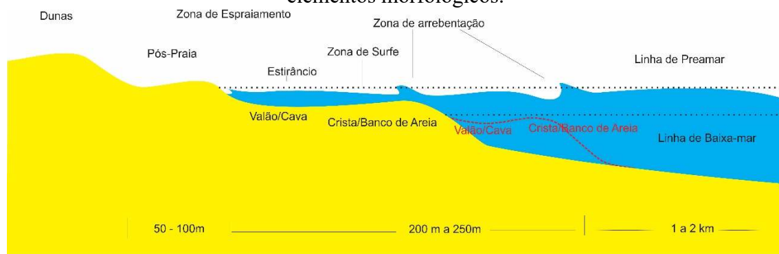
Figura 1 - Perfil generalizado de uma praia apresentando suas divisões e os principais elementos morfológicos.
