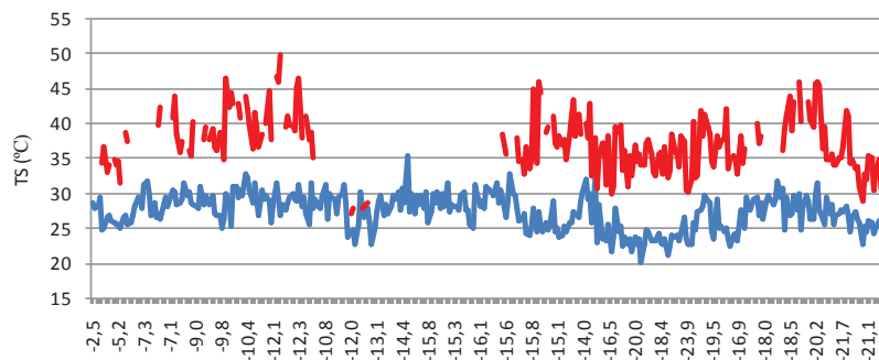
Figura 6 – Gráfico das distribuições das médias termais de superfície para a classe pastagem, conforme distribuição latitudinal. A cor azul representa a temperatura no mês de maio e a cor vermelha a temperatura no mês de setembro. Elaboração própria.
