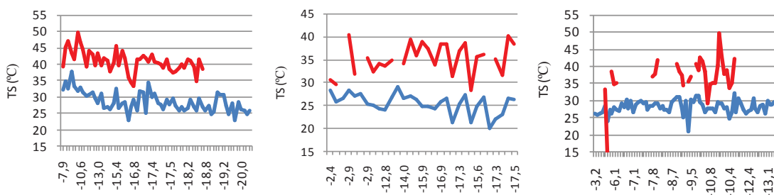
Figura 6 – Gráfico das distribuições das médias termais de superfície para a classe pastagem, conforme distribuição latitudinal. A cor azul representa a temperatura no mês de maio e a cor vermelha a temperatura no mês de setembro. Elaboração própria.
