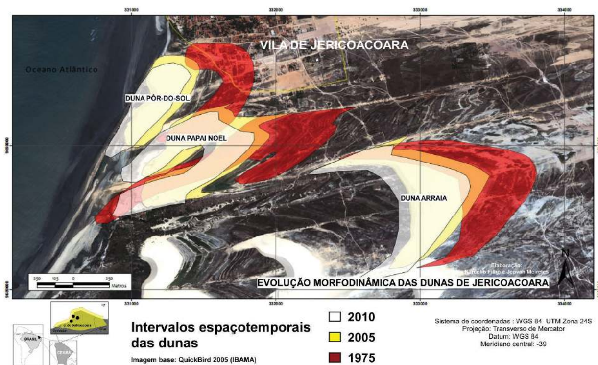
Figura 3 - Dunas barcanas e barcanóides de morfologias complexas devido dinâmica de transporte associada à incorporação de outras dunas durante a migração das maiores. Evidenciar relações com os demais sistemas ambientais diante da faixa de deslocamento. Verificar que a DPS chegou à faixa de praia.
