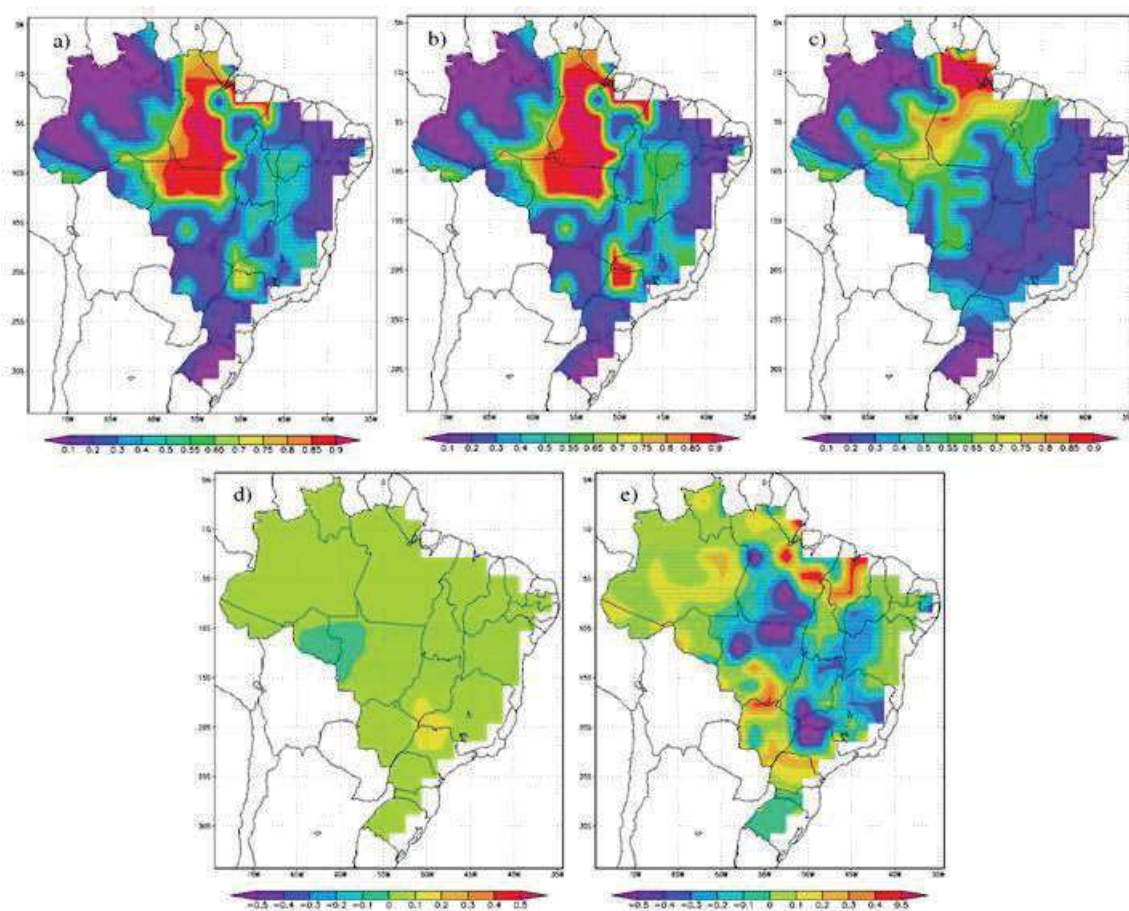
Figura 12 - a) Índice de Setzer (IS) para o clima e vegetação atual para setembro, b) IS para o clima futuro e vegetação atual para setembro, c) IS para simulações futuras de clima e vegetação para setembro; d) são as anomalias entre b) e a); e) são as anomalias entre c) e a).
