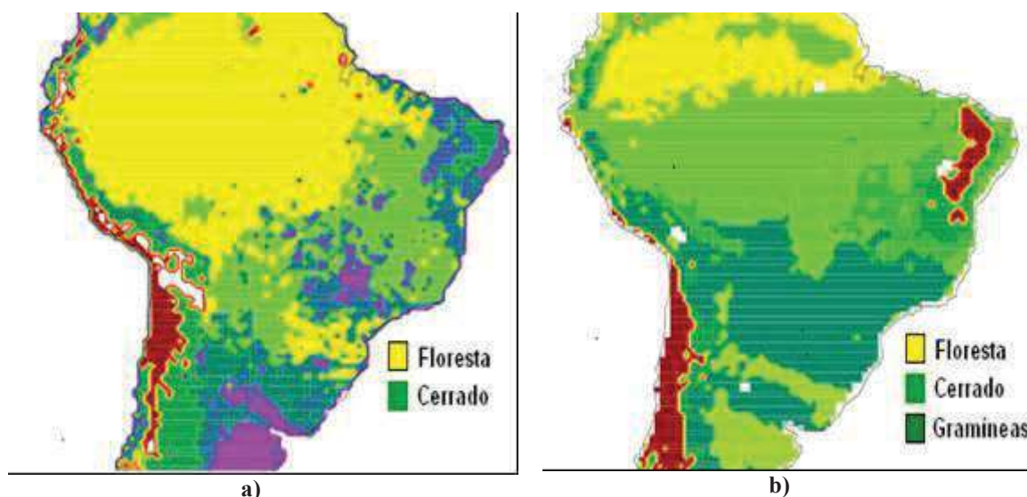
Figura 4 - a) Distribuição da vegetação atual na América do Sul (AS); b) Distribuição da vegetação prevista para o futuro na AS.
