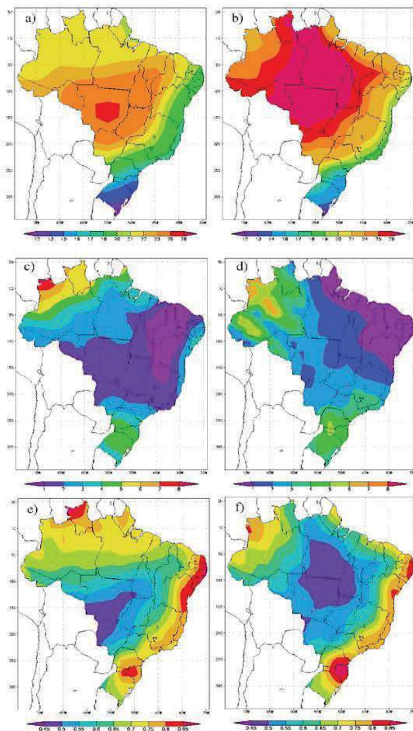
Figura 1 - Climatologia no período de junho a outubro, média dos anos 1980 a 2000.
