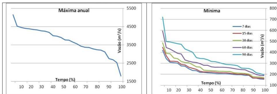
Figura 3 – Vazões Médias Diárias: Máxima Anual e Mínima da Bacia do rio Ivaí - PR. (1985-2012)
