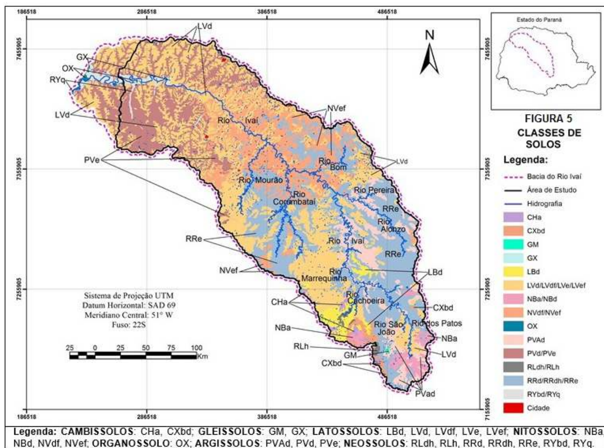
Figura 5 – Mapa de solos.
