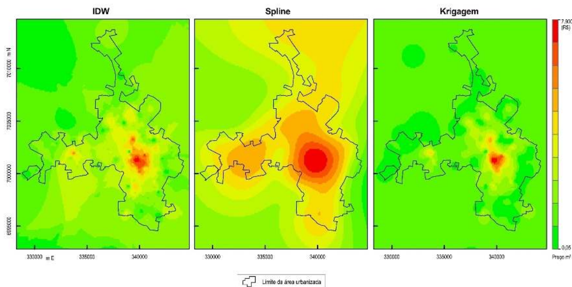
Figura 2 – Diferentes interpolações espaciais para a variável preço do metro quadrado de terreno.
