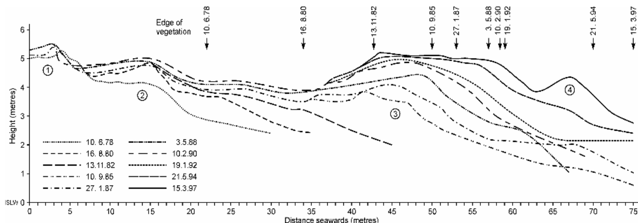
Figura 2: Perfis de Myall Lakes (da direita para a esquerda, os termos em inglês significam: nível médio do mar, altura em metros, limite de vegetação, distância do mar em metros).
