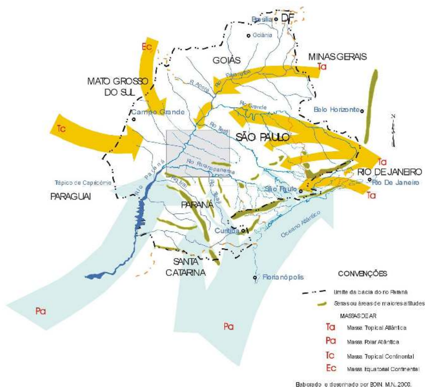
Figura 3 - Ação das massas de ar que influenciam o clima no Oeste Paulista e a área de estudo.
