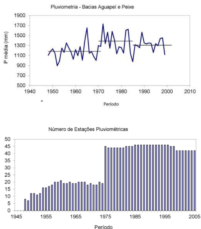
Figura 4 - Precipitação total anual média na área das bacias dos rios Aguapeí e Peixe, Oeste Paulista. A) Variação interanual e média dos períodos identificados; B) número de estações avaliadas.
