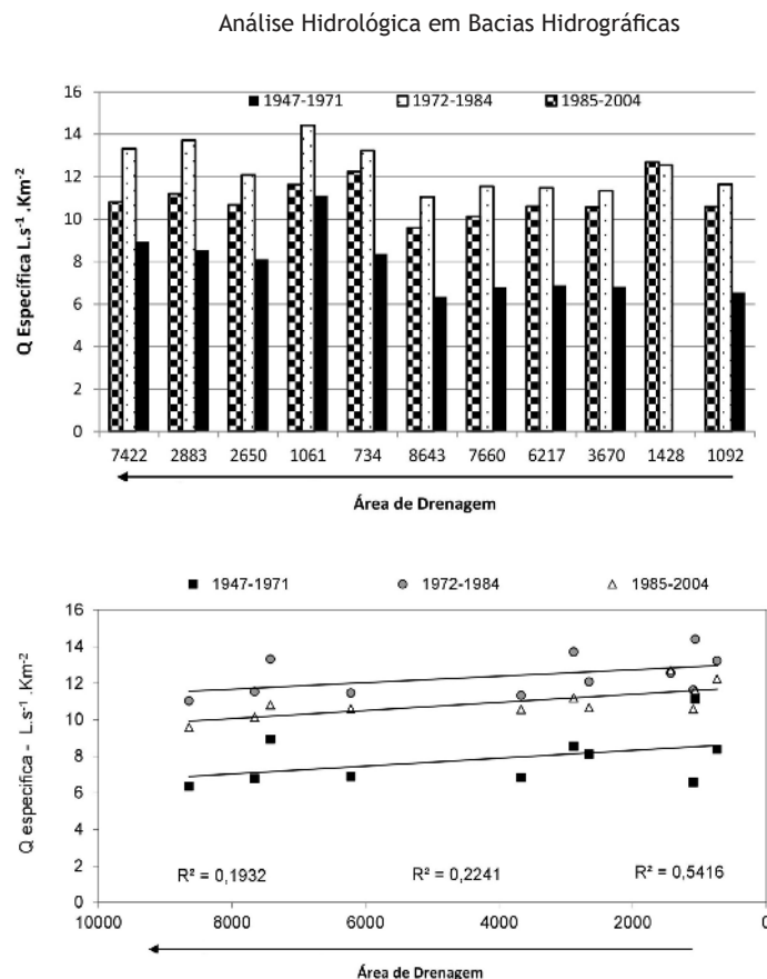
Figura 11 - Representação gráfica da variação temporal e espacial da vazão específica média nas bacias dos rios Aguaípe e Peixe. Fonte: Rocha & Andrade (2015).
