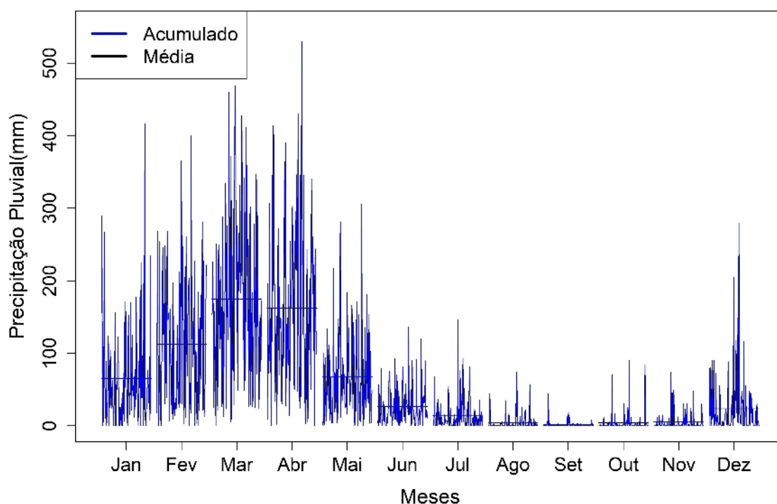
Figura 2 - Variabilidade intramensal com as respectivas médias da precipitação pluvial acumulada para Caicó, RN. Período:1911 a 2017.
