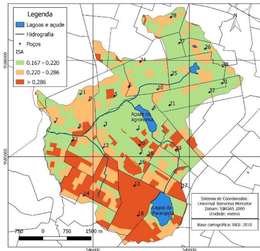
Figura 4 – Mapa de Índice de Saneamento Ambiental
