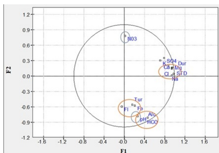
Figura 6 – ACP da qualidade da água dos poços no período chuvoso. Legenda: Tur - turbidez; FI - fluoreto; Fe - ferro; Alc - alcalinidade; K - potássio; Ca - cálcio; Mg -magnésio; Dur - dureza; Na - sódio; \text{NO}_3 - nitrato; \text{SO}_4 -sulfato; STD - sólidos totais dissolvidos.
