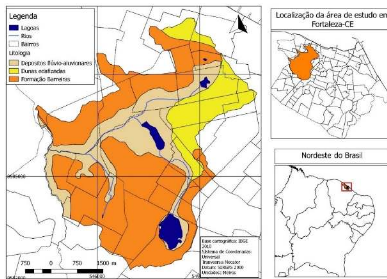
Figura 1 – unidades litológicas da área de estudo
