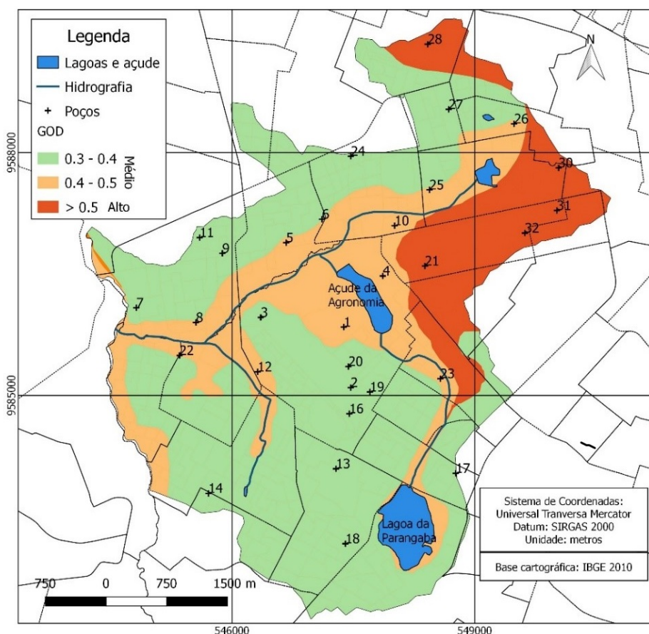
Figura 3 – Mapa de Vulnerabilidade aquífera GOD
