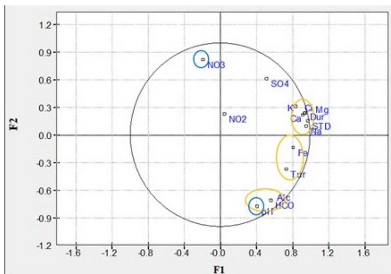
Figura 7 – ACP da qualidade da água dos poços no período seco. Legenda: Tur - turbidez; F1 - fluoreto; Fe – ferro; Alc - alcalinidade; K – potássio; Ca – cálcio; Mg –magnésio; Dur – dureza; Na – sódio; \text{NO}_3^- – nitrato; \text{SO}_4 –sulfato; STD – sólidos totais dissolvidos
