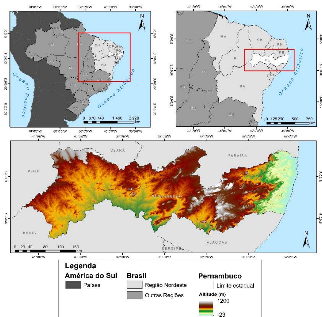
Figura1 - Mapa de localização e hipsometria da área de estudo (estado de Pernambuco). Fonte: Autores. Base de dados: Nasa Earth Data.
