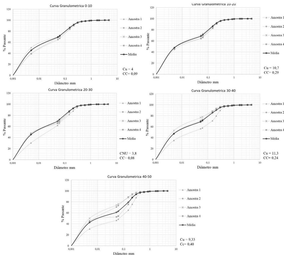
Figura 5 - Curvas Granulométricas do solo. *Cu-Coefficiente de Uniformidade; *Cc-Coefficiente de Curvatura. Fonte: Autores.
