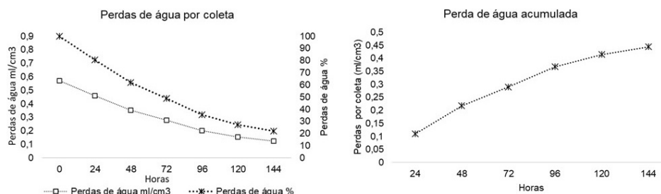
Figura 8 - Perdas de água por evaporação. Fonte: Autor.
